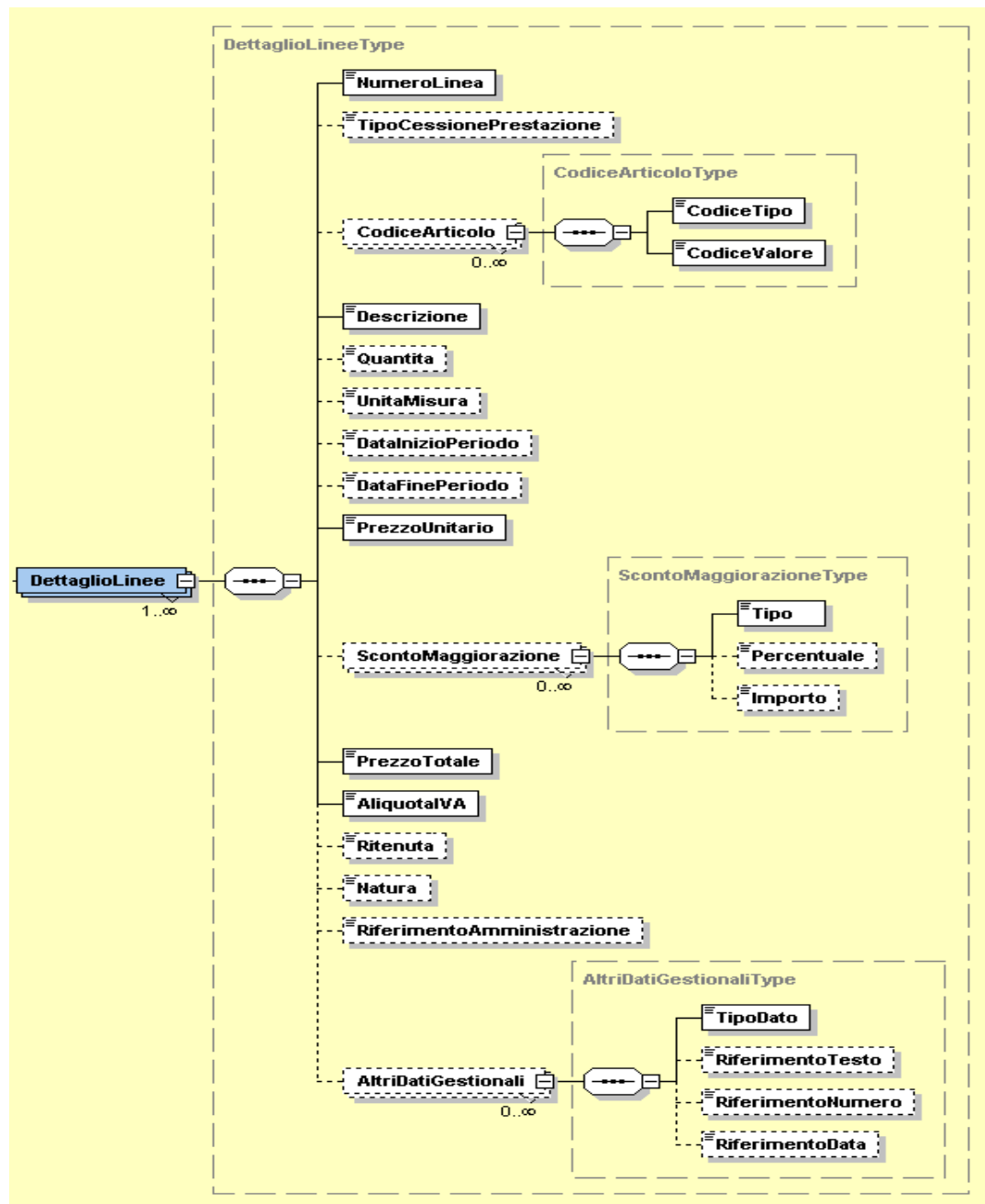
Figura 27: Elemento DettaglioLinee
