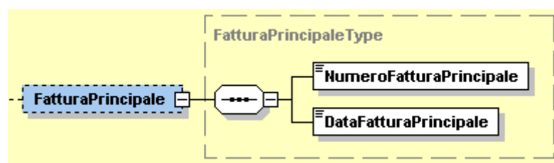
Figura 25: Elemento FatturaPrincipale
